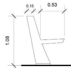
3 VISTA LATERAL ESC 1:50
