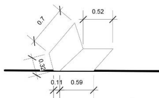
3 VISTA LATERAL ESC 1:50
